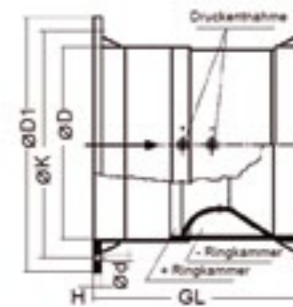
Kurz-Venturirohr Flanschversion
